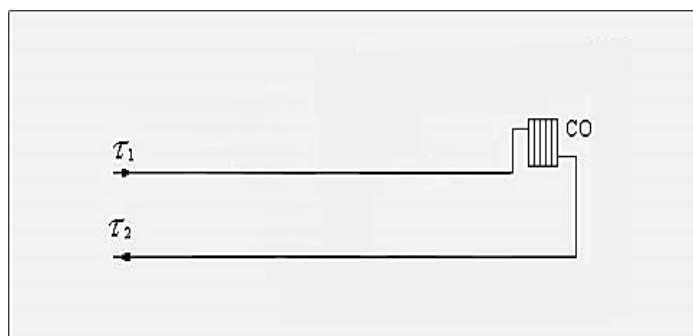
Рисунок 1 - Схема подключения потребителей к двухтрубной тепловой сети (при наличии внутренней системы отопления), зависимое присоединение, без смешения
